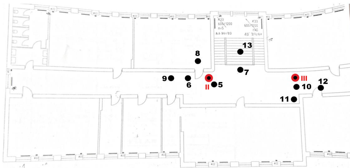
Rys. 1b: Plan rozmieszczenia punktów pomiarowych – I piętro kolorem czerwonym oznaczono lokalizację punktów dostępnych
