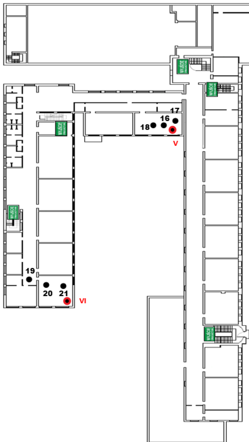
Rys. 1c: Plan rozmieszczenia punktów pomiarowych – II piętro kolorem czerwonym oznaczono lokalizację punktów dostępowych
