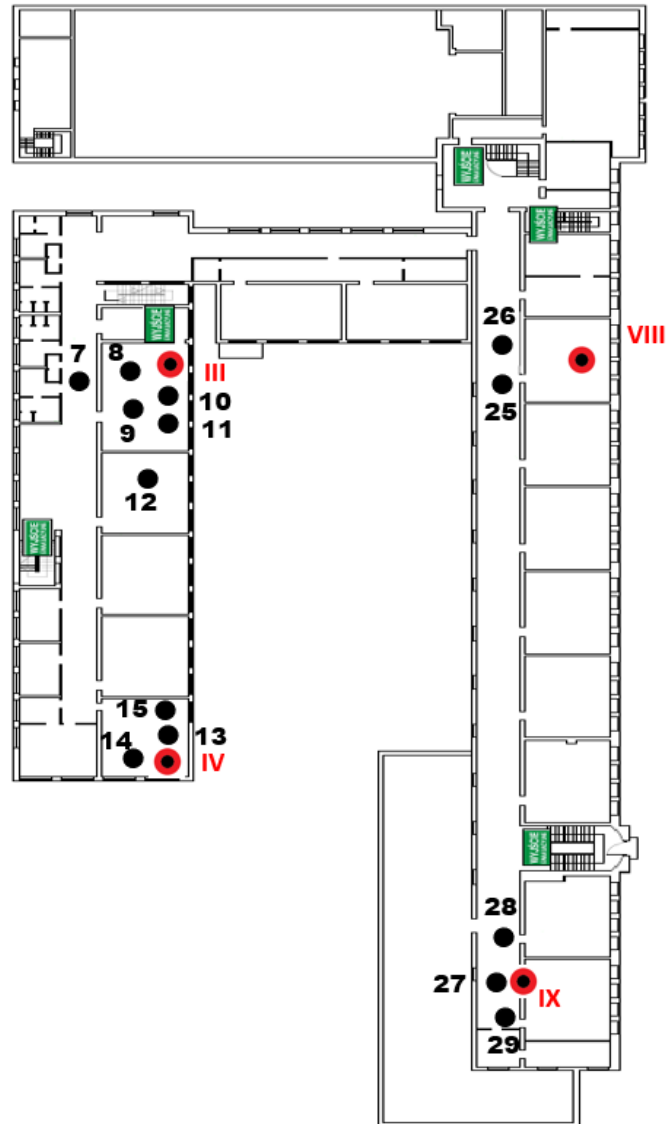
Rys. 1b: Plan rozmieszczenia punktów pomiarowych – I piętro kolorem czerwonym oznaczono lokalizację punktów dostępowych
